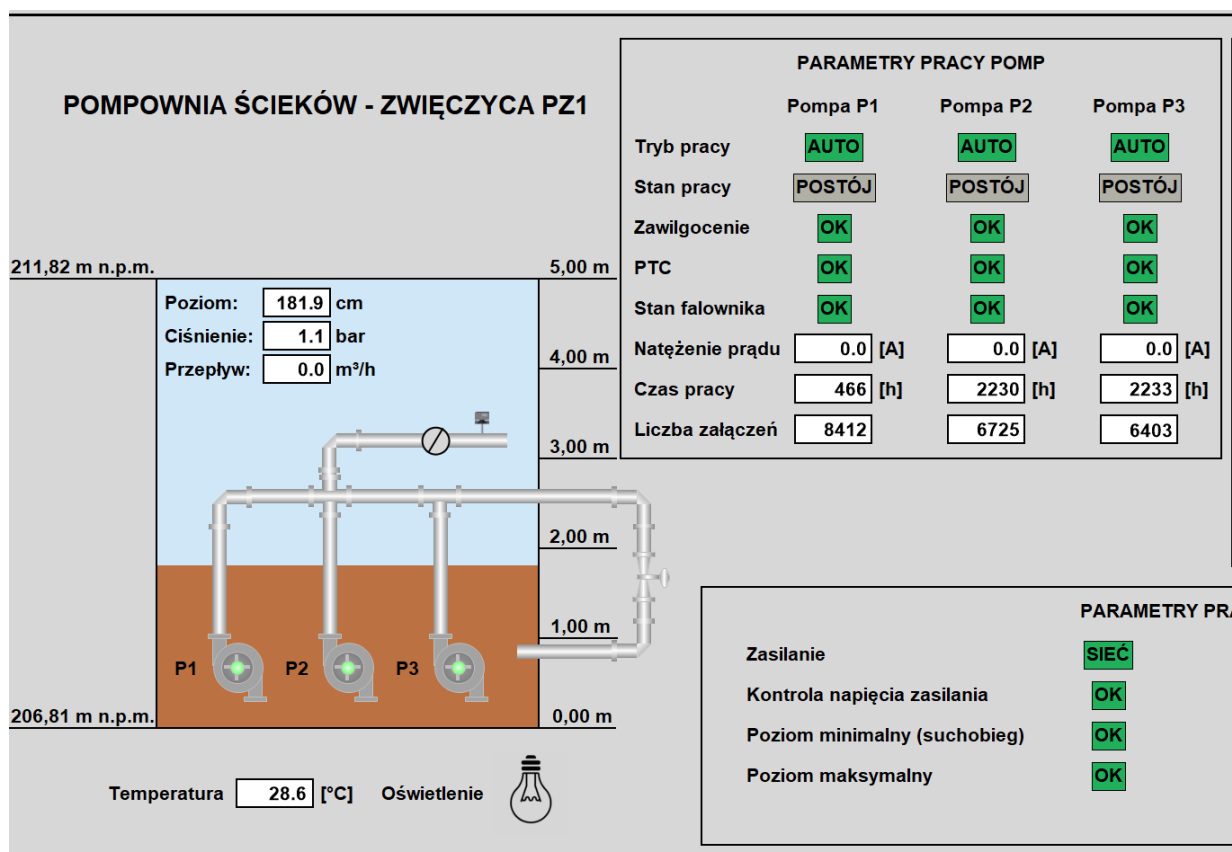
Pompownia ścieków Zwięczyca - schemat
