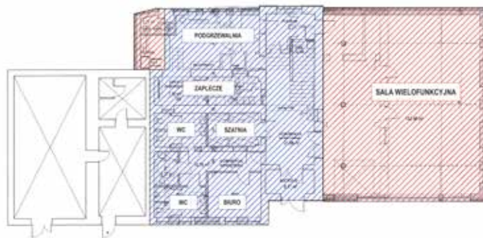
Schemat układu pomieszczeń Domu Kultury w Zarzeczcu
